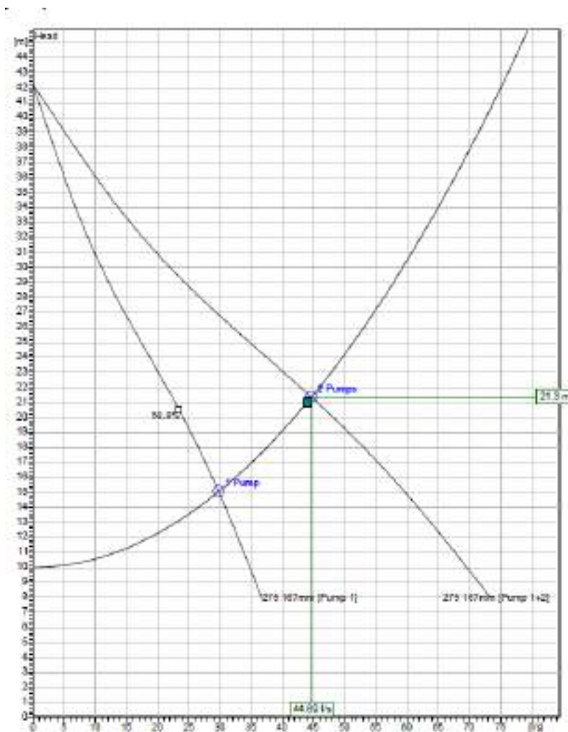
slika 3. Radni dijagram odabrane crpke Q = 30,00 \text{ l/s} i H = 15,00 \text{ m} u pojedinačnom i paralelnom radu
